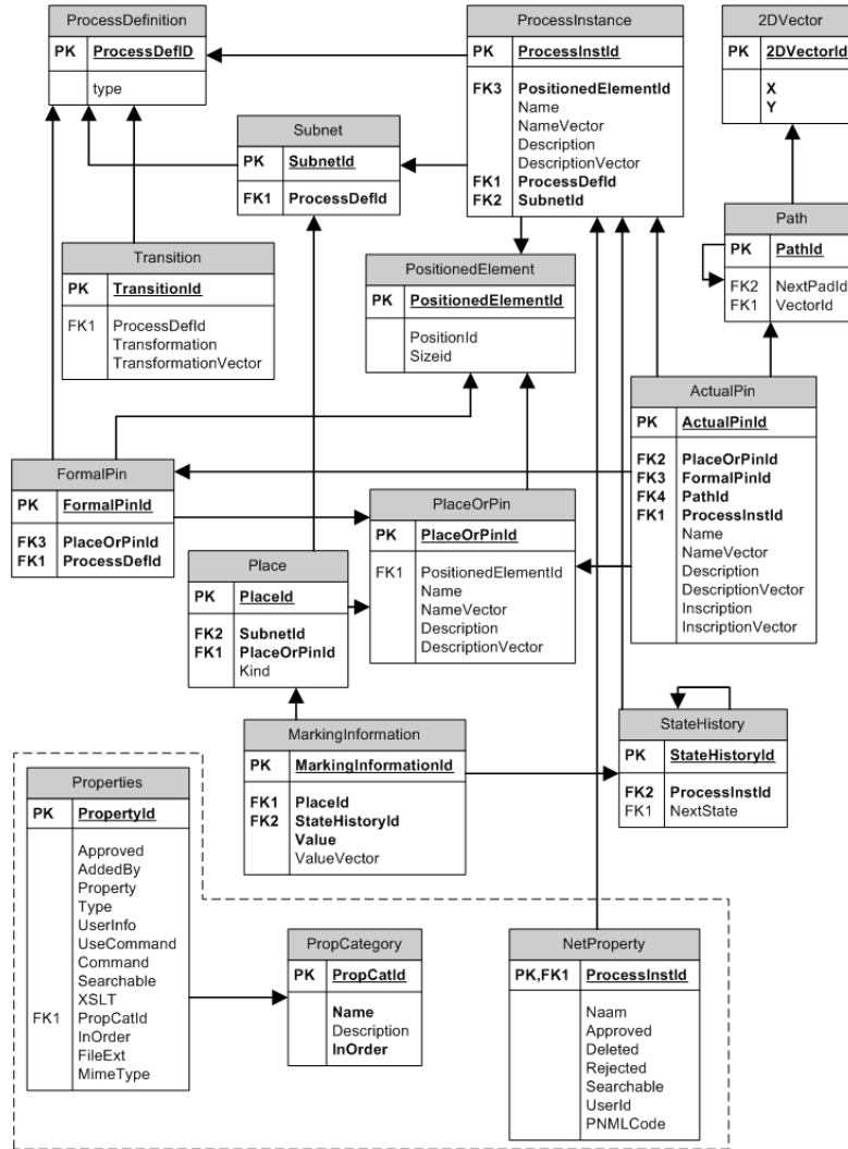
Fig. 3. Data schema of Petriweb
